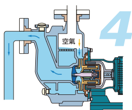
停止1(逆流狀態)
