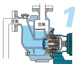
運轉前的靜止狀態
