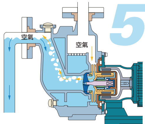
停止2 虹吸狀態(殘留水)
